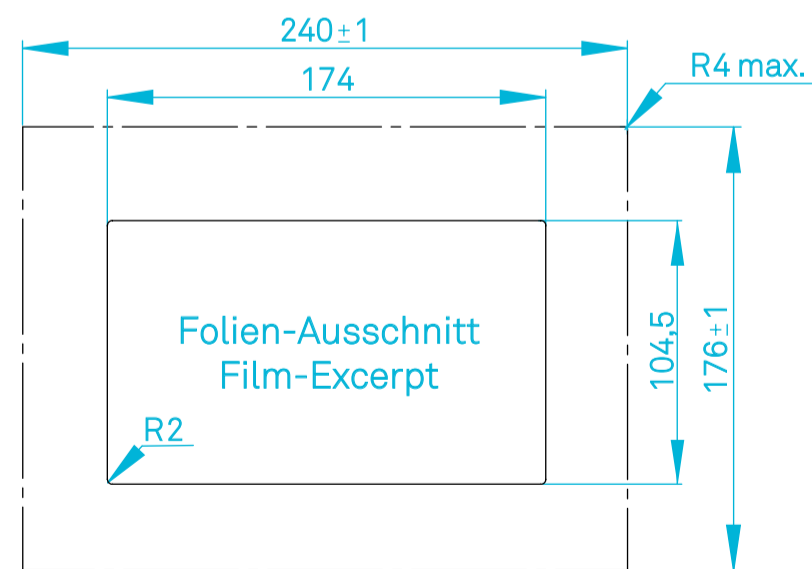
Einbau-Ausschnitt OPC7008 Mounting-Cutout OPC7008
