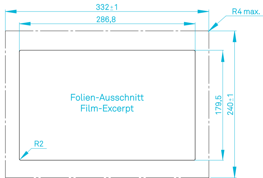
Einbau-Ausschnitt OPC7013 Mounting-Cutout OPC7013
