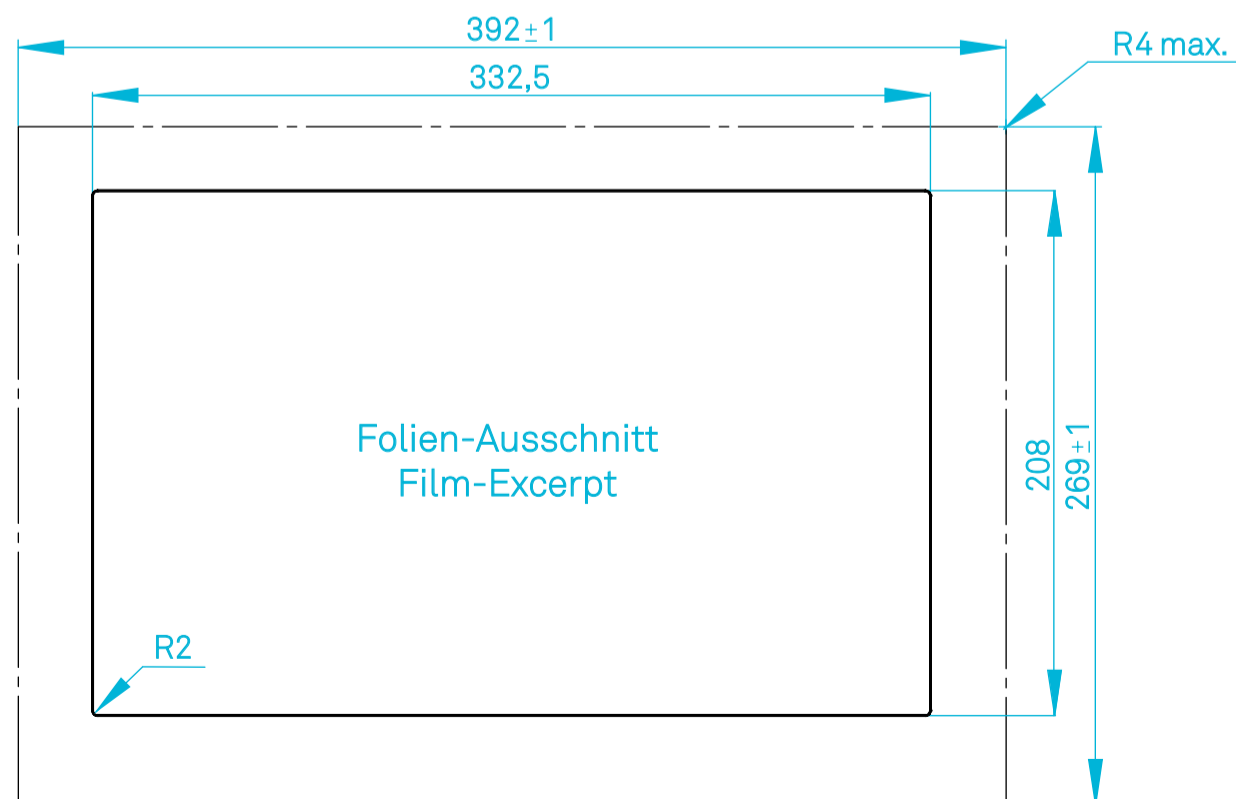
Einbau-Ausschnitt OPC7015 Mounting-Cutout OPC7015
